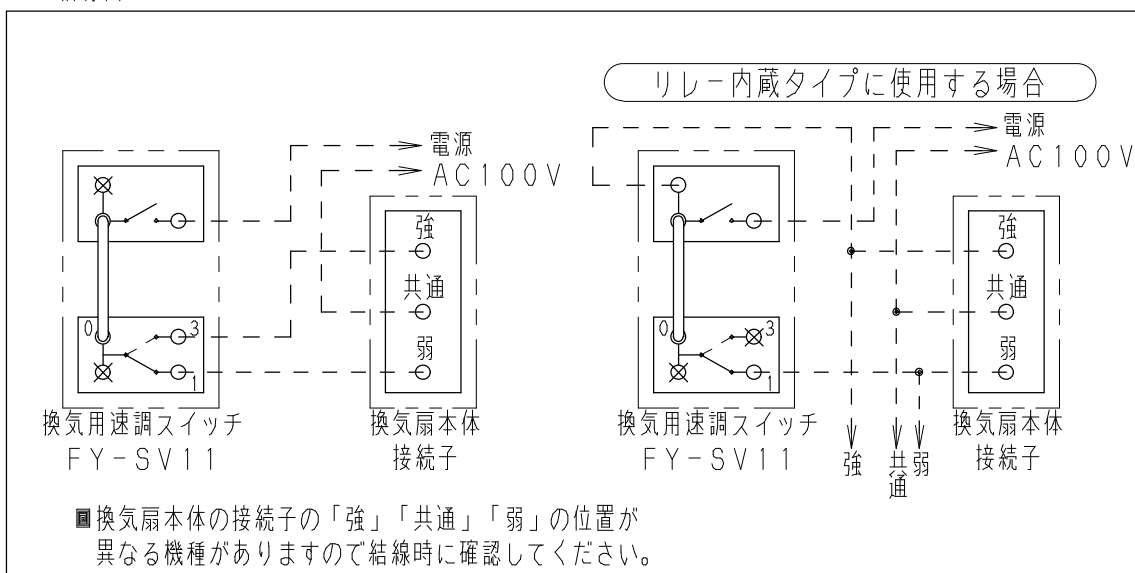
■ 結線図
